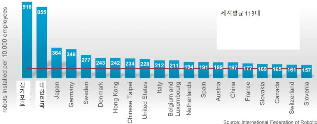
2019년 전 세계 산업용 로봇 밀도
